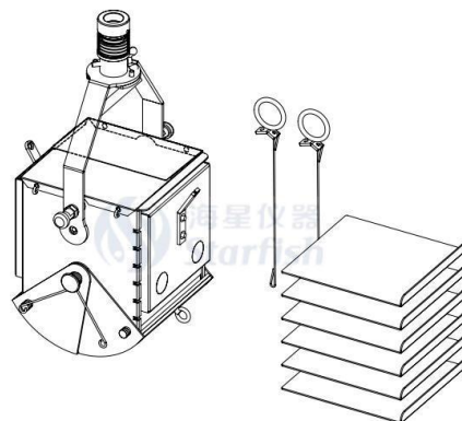
CNX-0002 箱式/分层箱式采泥器
